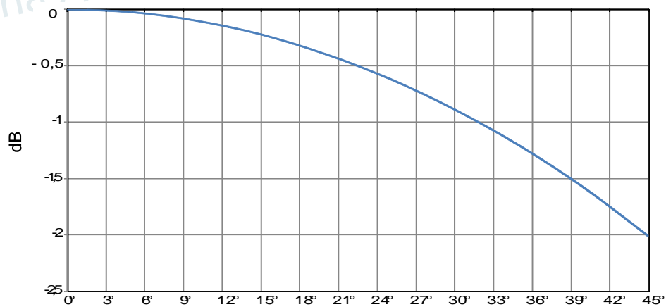
Diagrama de Elevación
