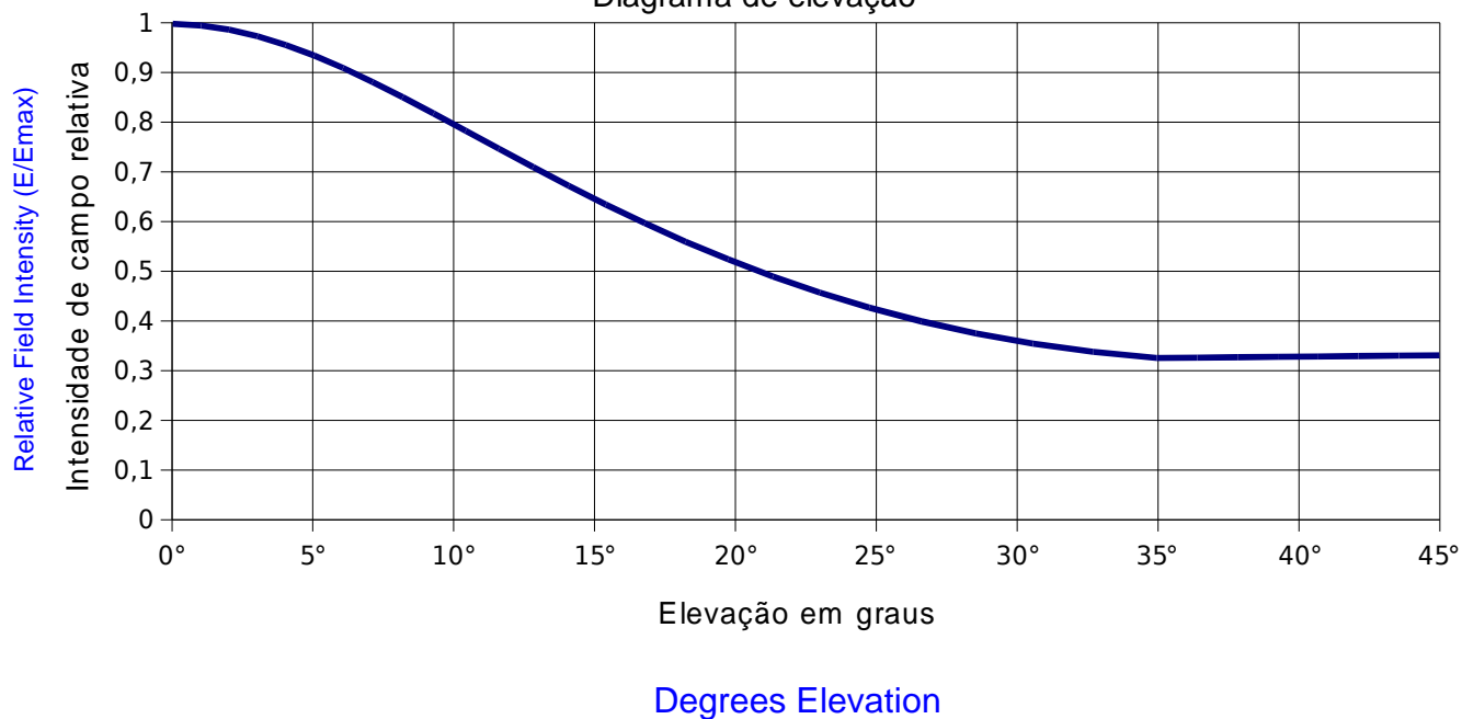
Plano Terra 2.5/8" Bobinada Diagrama de elevação
