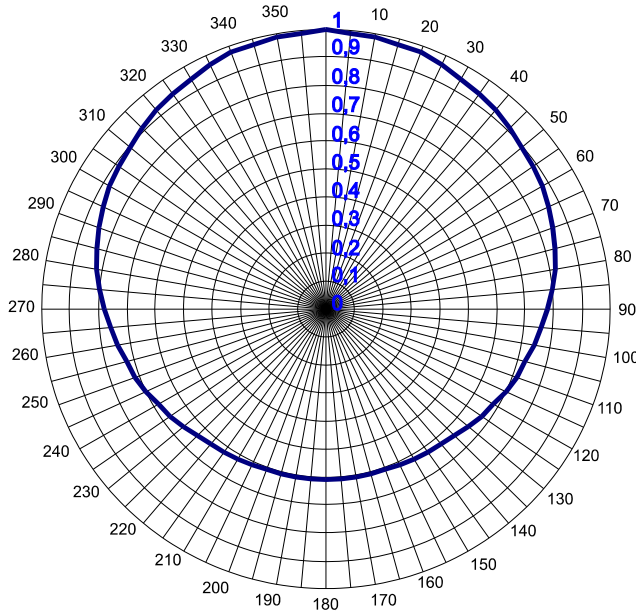
Diagrama de Elevação para 1 elemento
