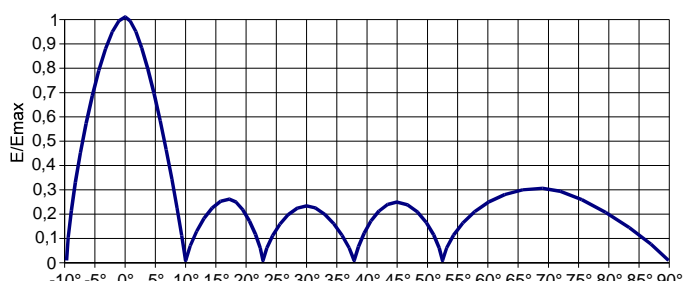
Diagrama de Elevação para 6 elementos
