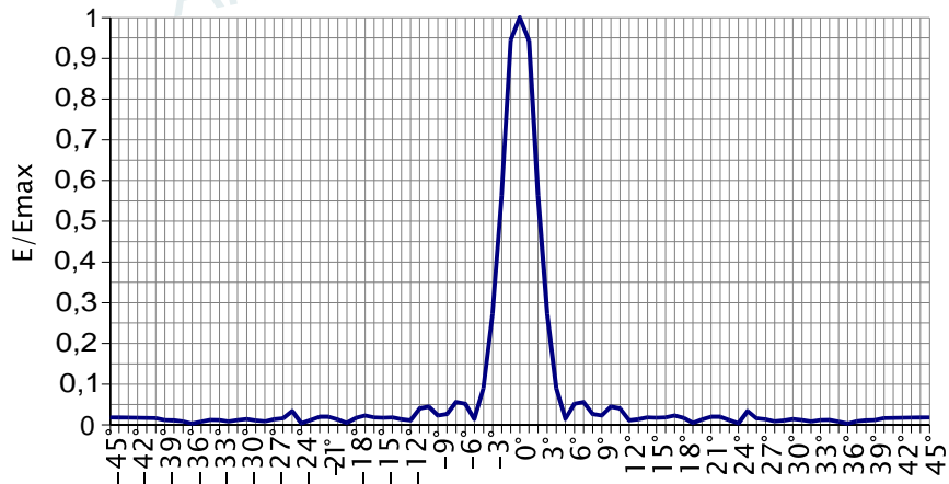
Diagrama polarização vertical
