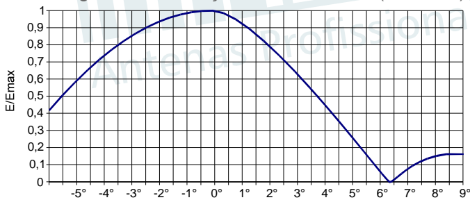
Diagrama de Elevação - Painel 8,5 dBi (6,35 dBd)
