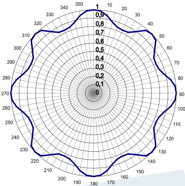
Diagrama de Azimute na polarização Vertical
